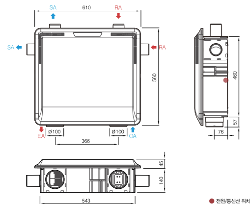
제품 치수(단위:mm)
